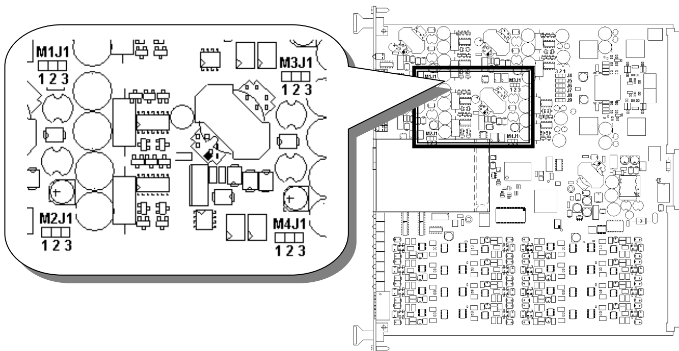
Рис.4.11 Вид стационарного устройства и конфигурационных перемычек дистанционного питания (ДП) по каждому источнику.
