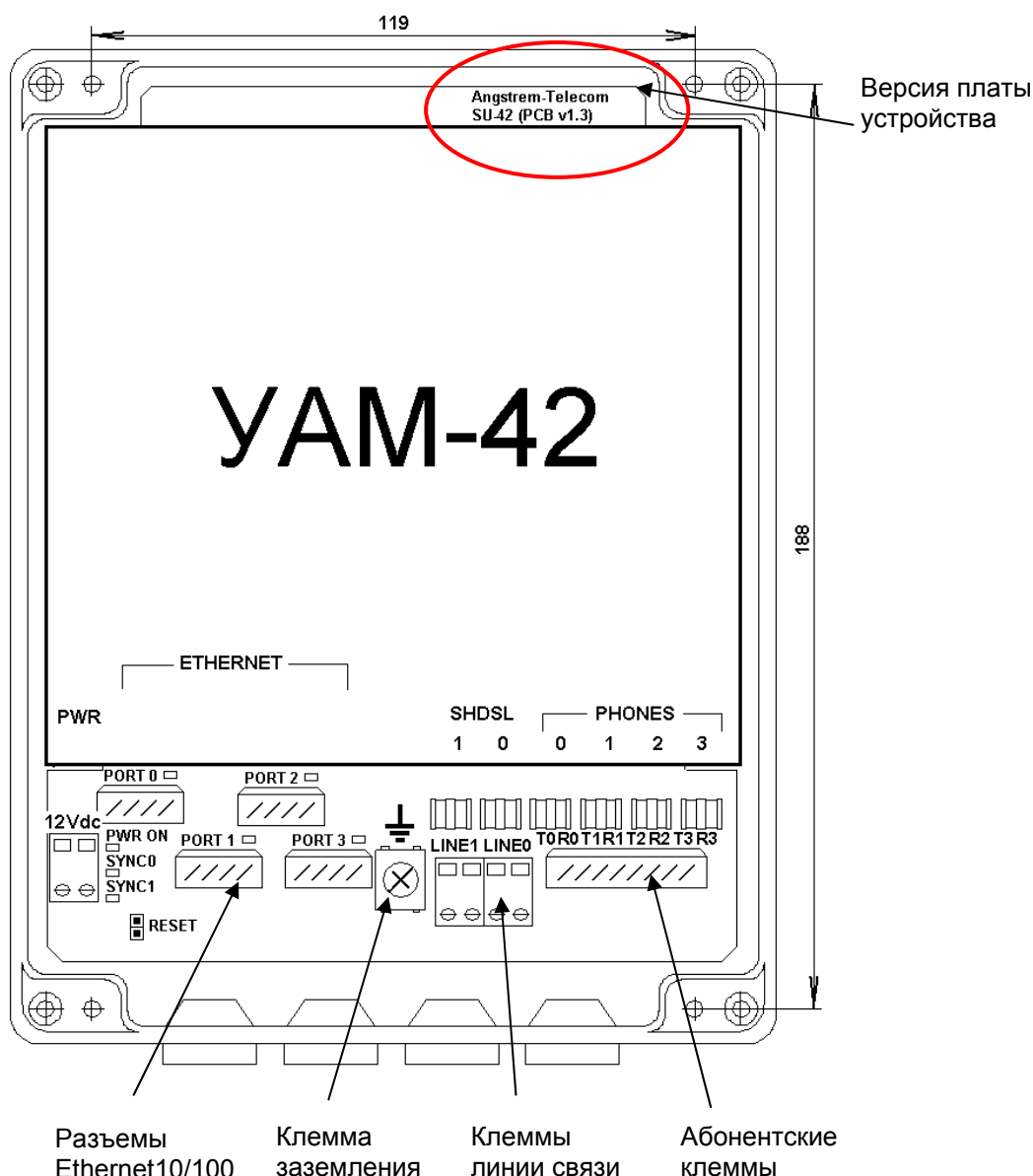
Рис.4.14 Назначение контактов абонентского устройства УАМ-42-4
