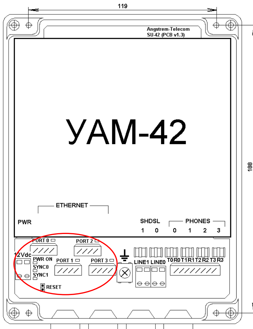
Рис 4.8. Индикаторы абонентского устройства
