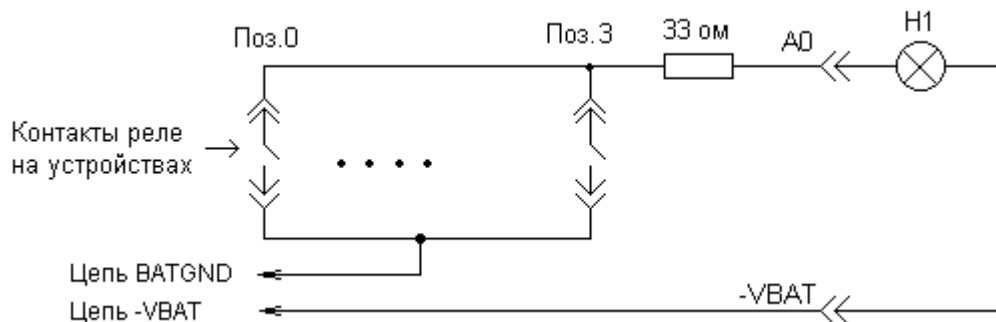
Рис.4.16 Схема цепей аварийной сигнализации и пример подключения лампы световой сигнализации H1 на каркасе K4.
